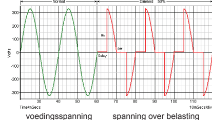
Fase aansnijding (leading edge) principe
