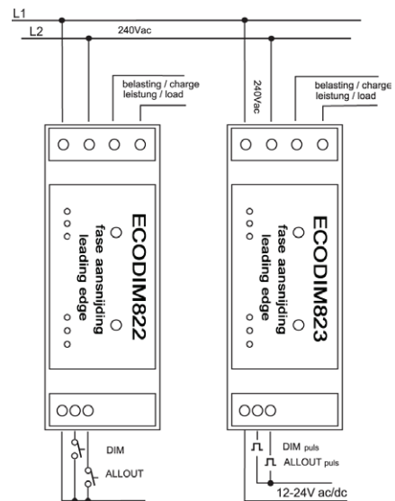
Fase aansnijding (leading edge) principe
